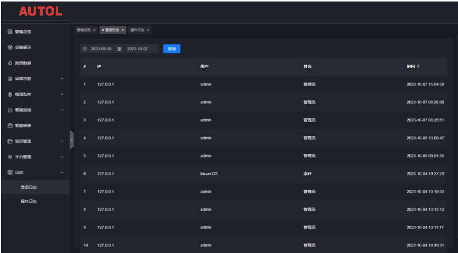
Login log
